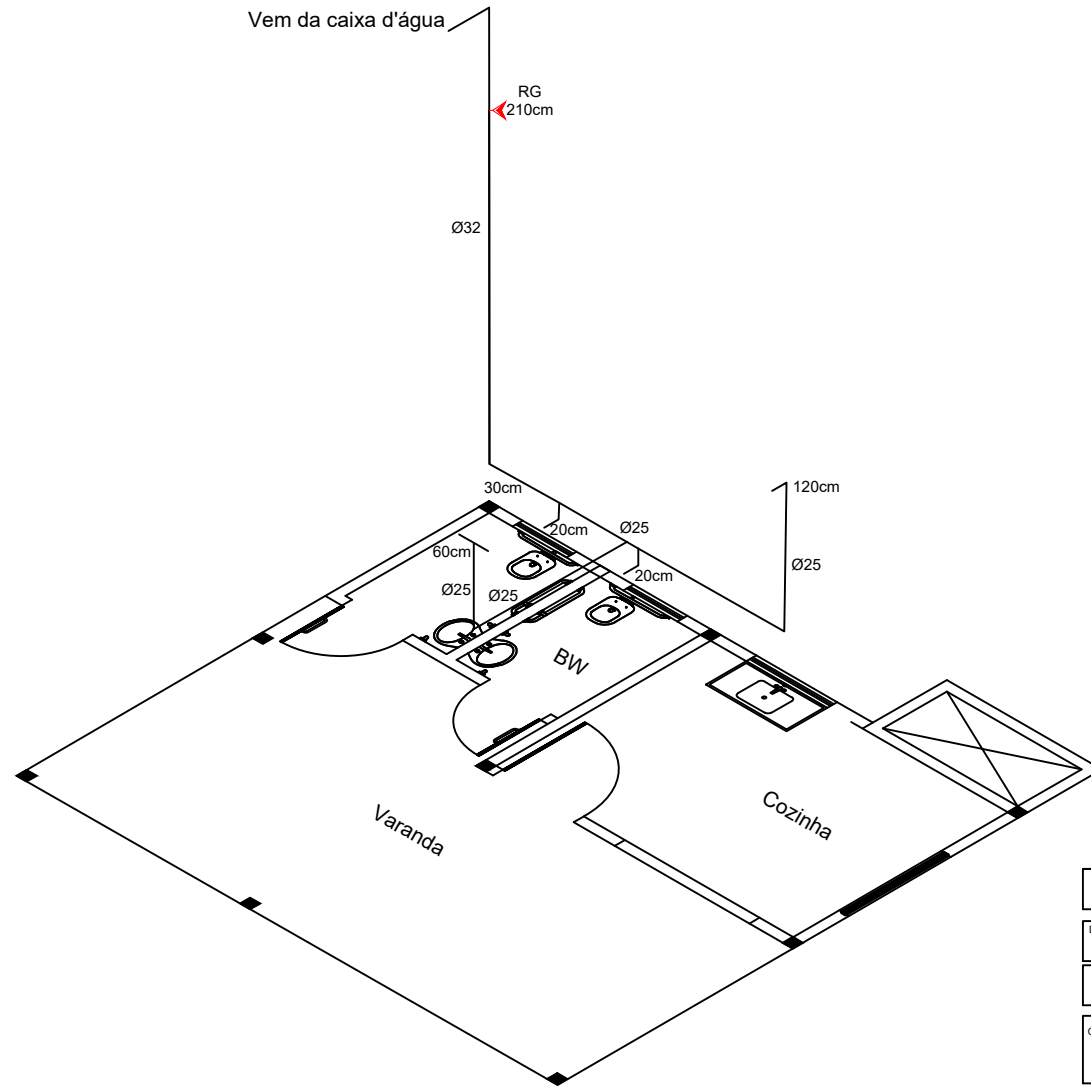
INSTALAÇÕES HIDRÁULICAS
