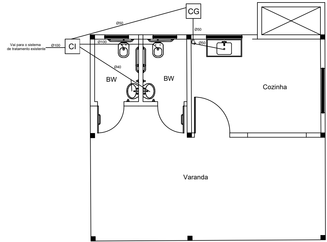
INSTALAÇÕES SANITÁRIAS
