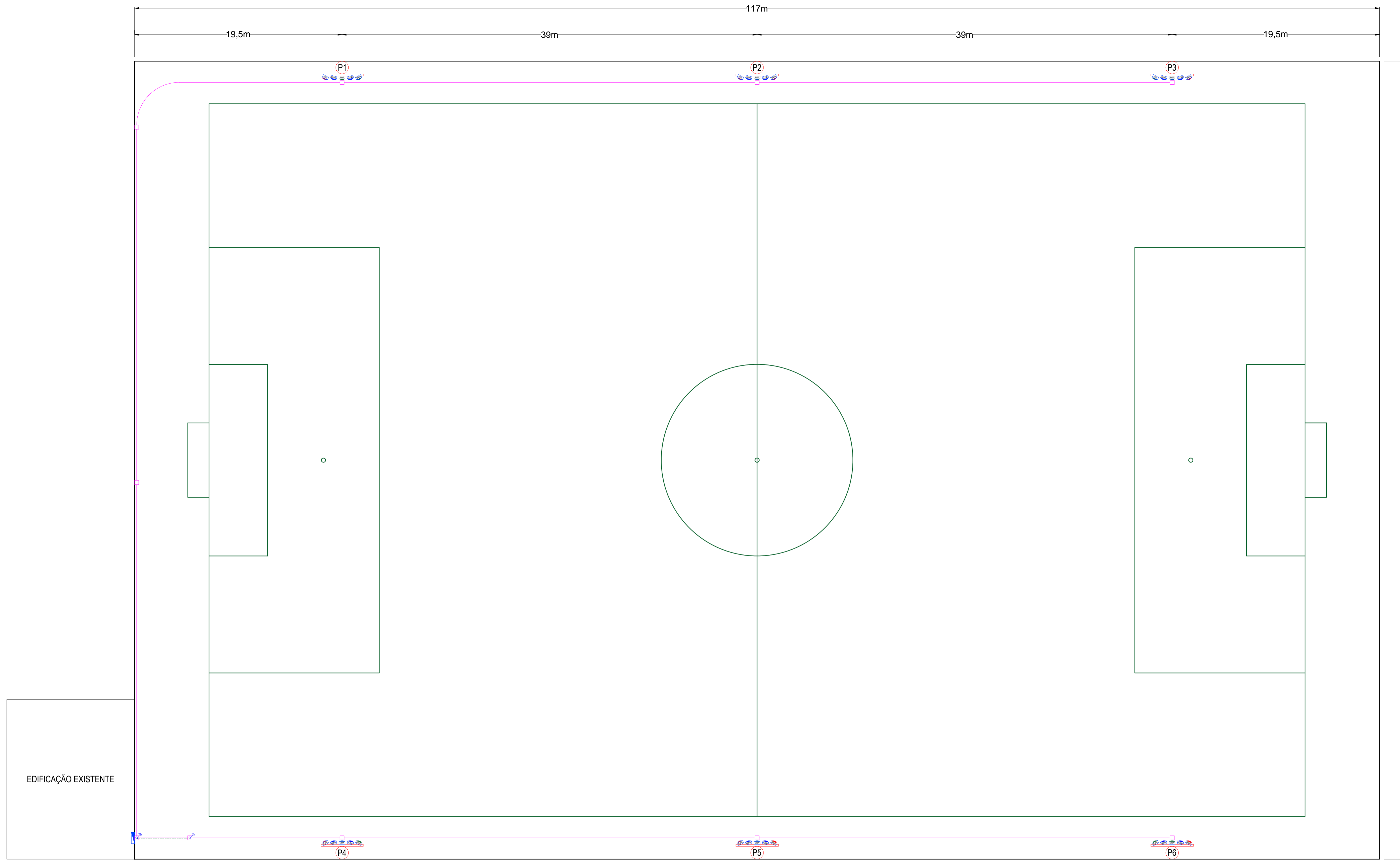
① PLANTA BAIXA - ILUMINAÇÃO ESTÁDIO ESCALA: 1:200
