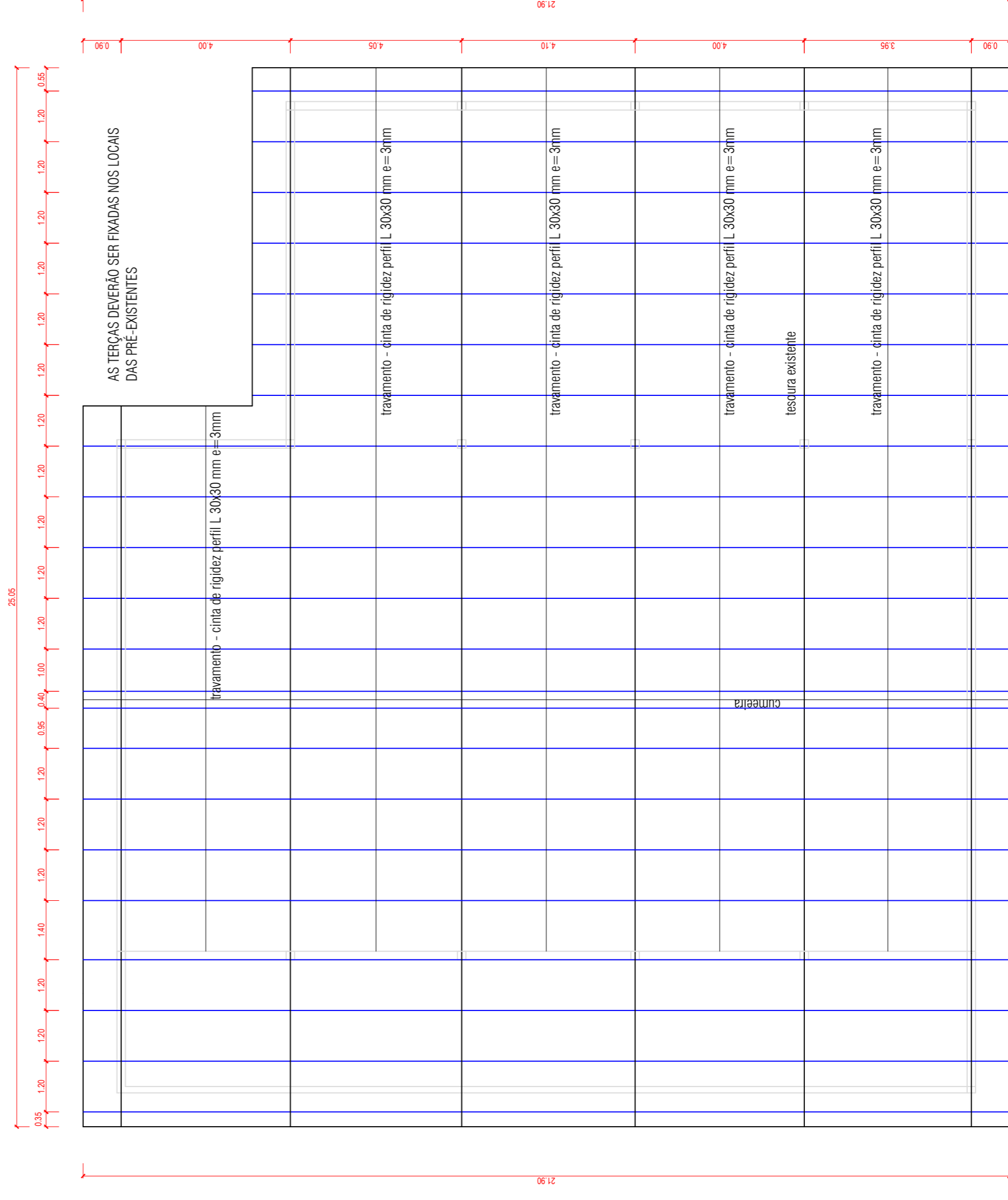
PLANTA DE LOCAÇÃO DE TERÇAS E TELHAS
